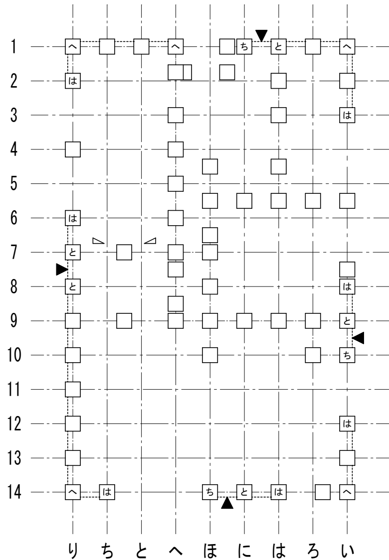
1 階柱壁伏図
